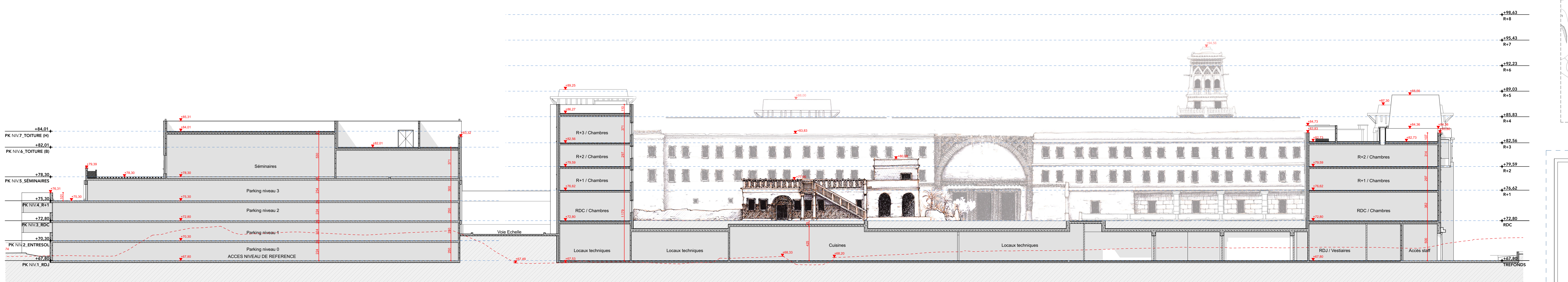
I Coupe Facade I Hôtel + Parking 1:200
